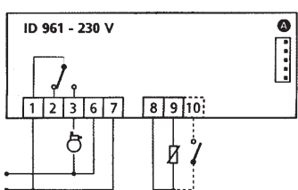
ID 961/A NTC
