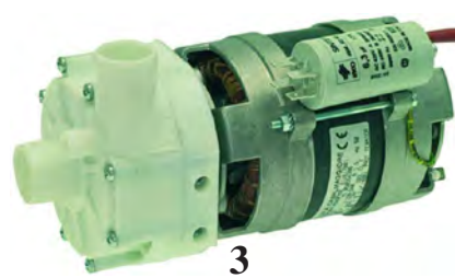
Huuhtelup.1010C 230V 100L/min. 0,28 kW - 1,5A - 6,3 uf Sisään 25 mm ulos 25mm ZANUSSI
